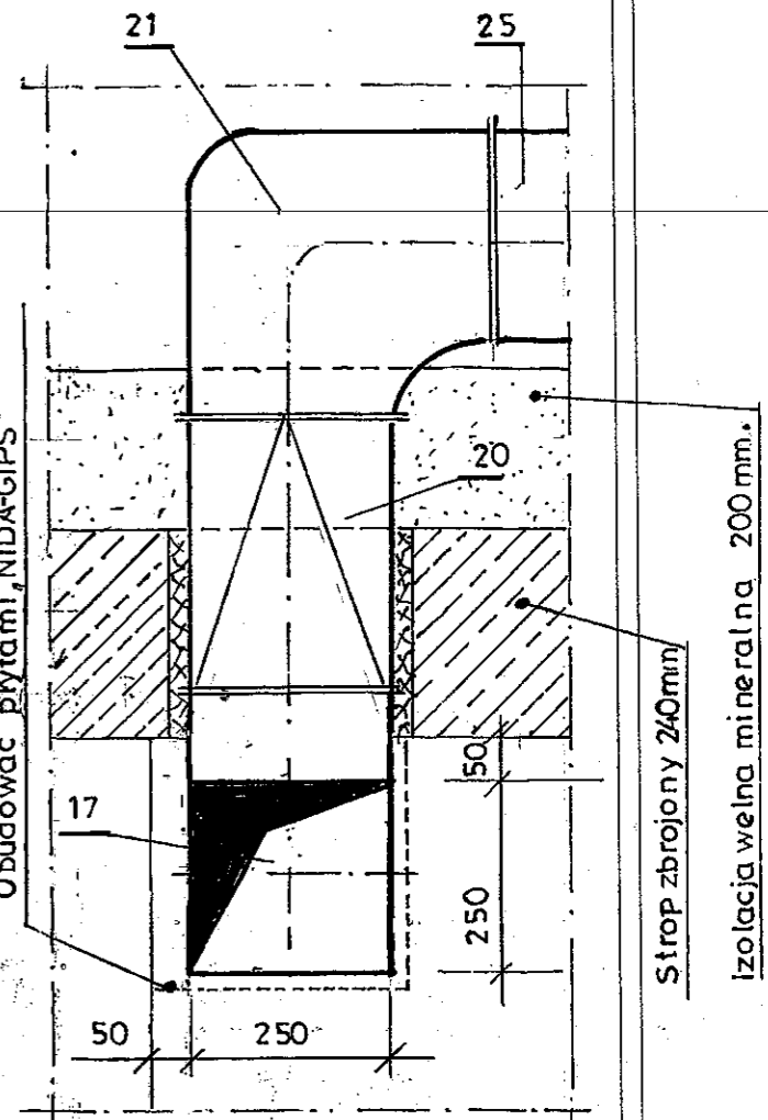
Przekrój E-E • 1:10 •
